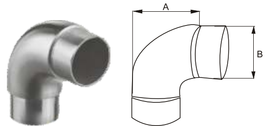
MV-005 TORUPÖLV
