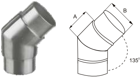
MV-002 TORUPÖLV 45°
