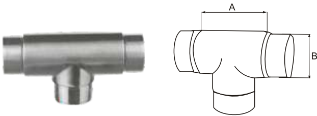
MV-010 T-ÜHENDUS
