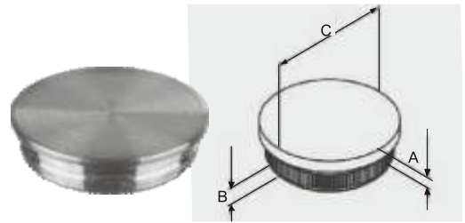
MV-008.1 OTSAKINNIS
