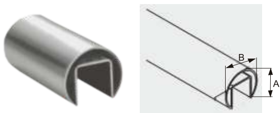
MV-040 U-PROFIL
