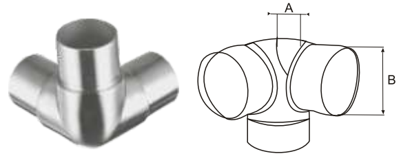
MV-017 T-ÜHENDUS
